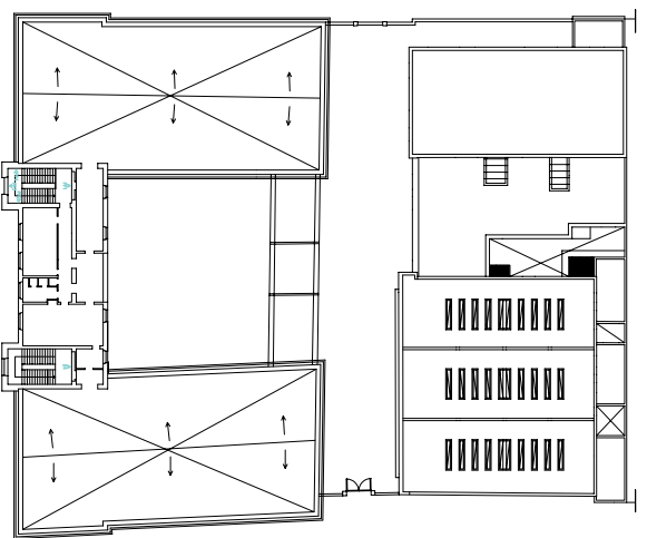
PIANTA PIANO TERZO scala 1:100
